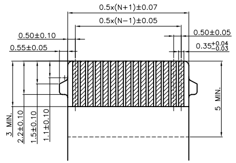
RECOMMENDED FPC DIM. RECOMMENDED FPC DIM.
